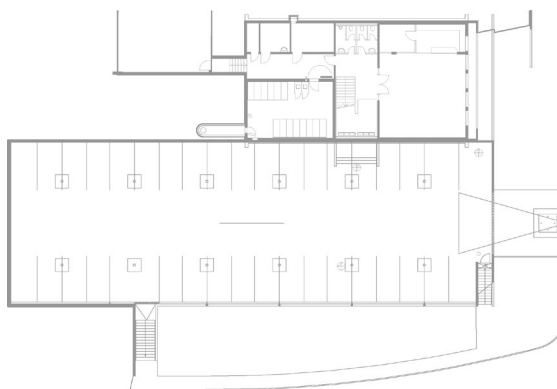
Plan du sous-sol
